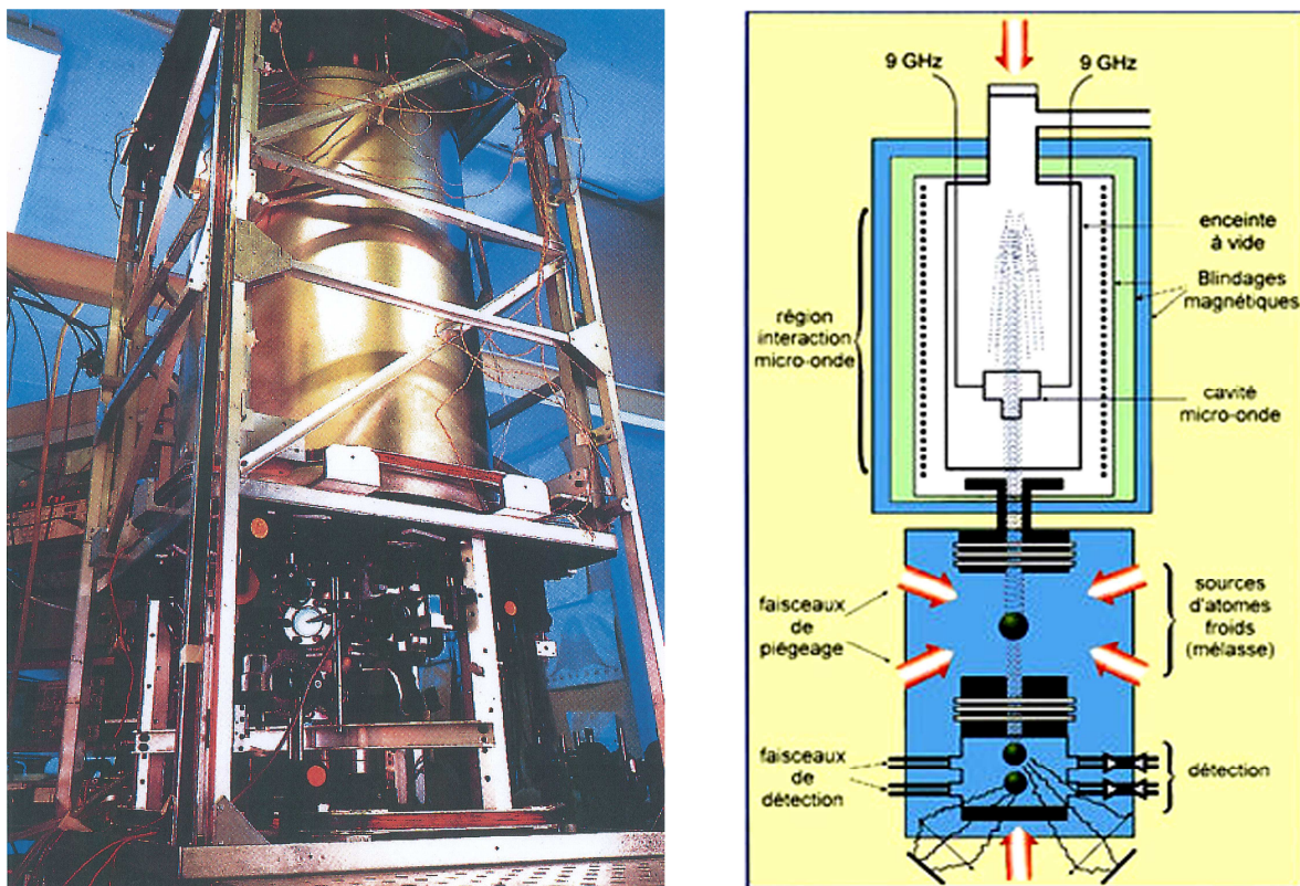
Figure 1: Fontaine atomique du BNM-LPTF à l'Observatoire de Paris; schéma du tube horloge (à droite) et photo de la fontaine F01 (à gauche). @ BNM-LPTF, Observatoire de Paris
