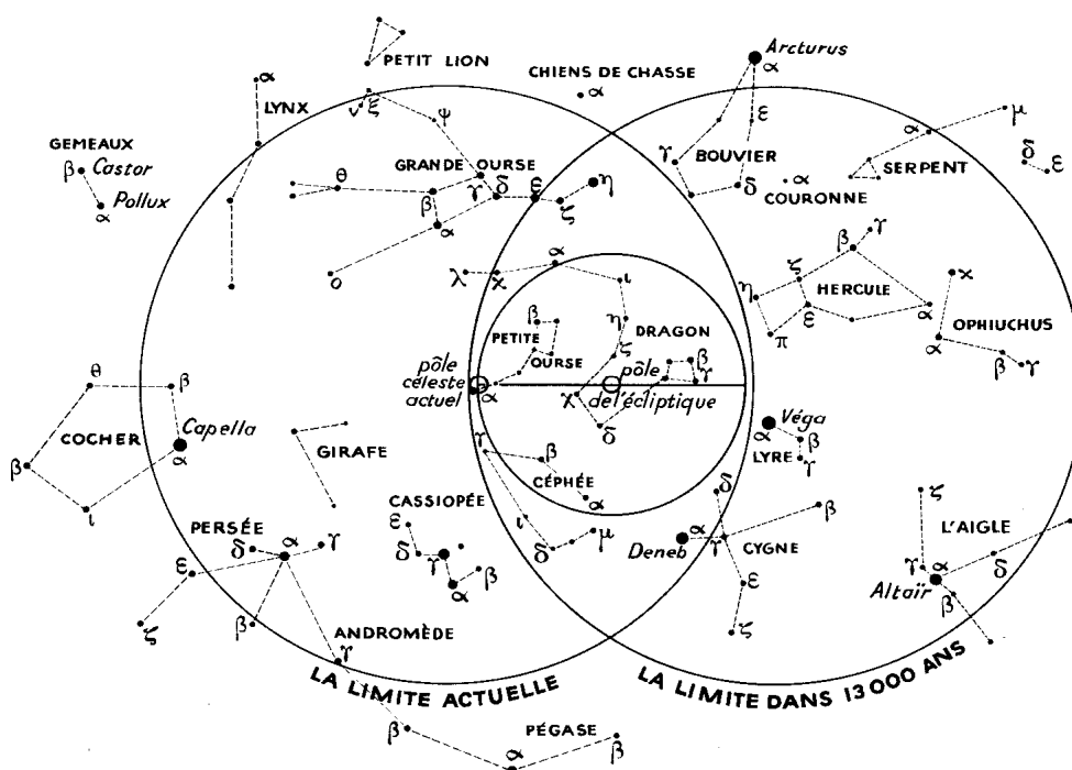
Figure 1 : Constellations boréales visibles à nos latitudes dans les deux configurations à 13000 ans d'intervalle (extrait de " L'Astronomie populaire " de Flammarion)
